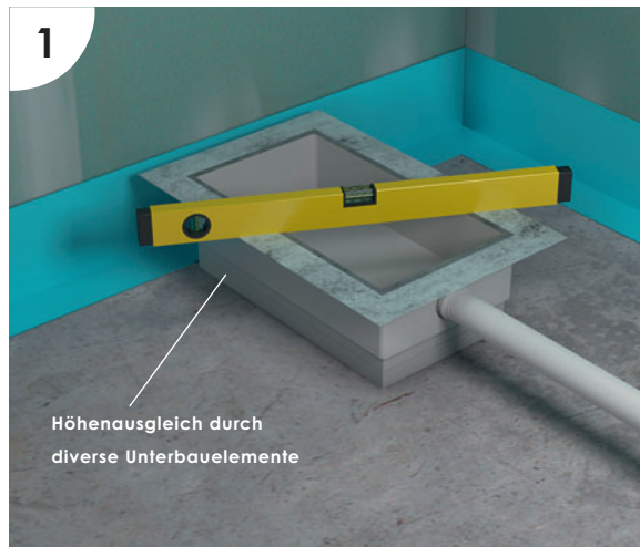
AUSRICHTEN DER ABLAUFBOX
