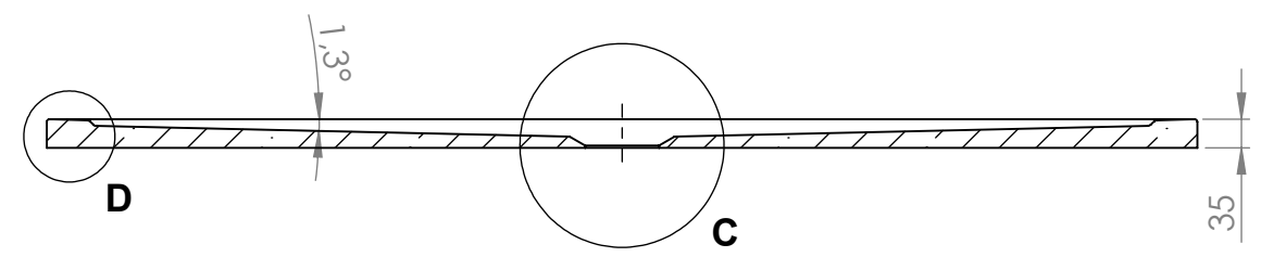
SECTION A-A
