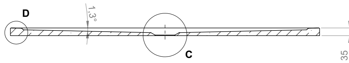
SECTION A-A
