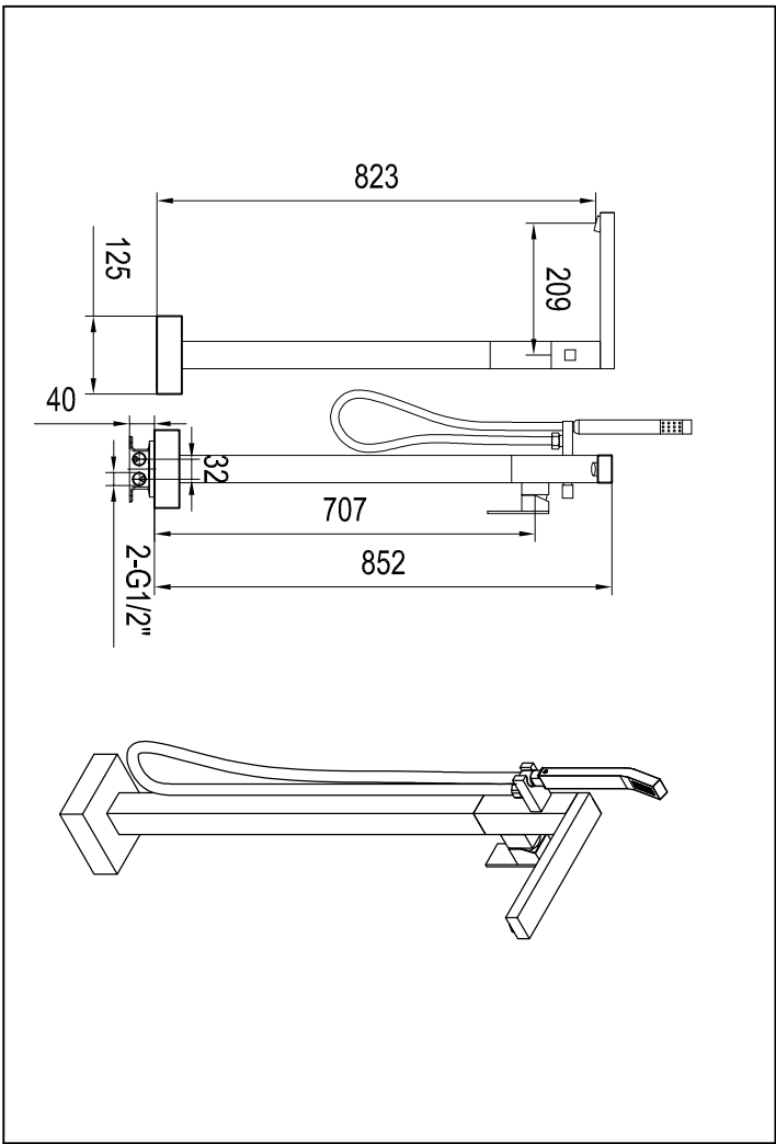
Technische Zeichnung/Explosionszeichnung
