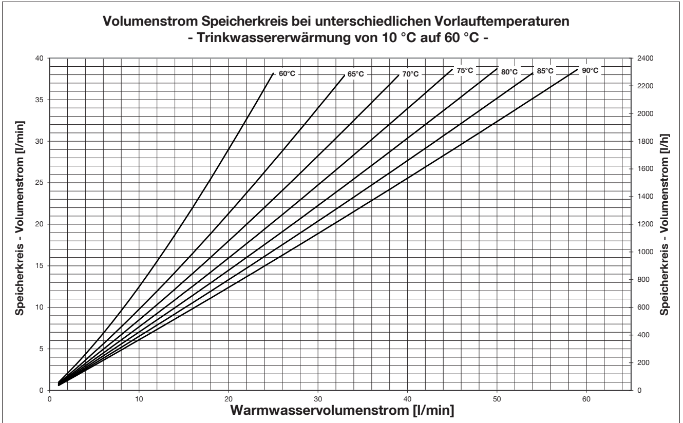
Abb. 45: Volumenstrom Speicherkreis - Trinkwassererwärmung auf 60 °C
