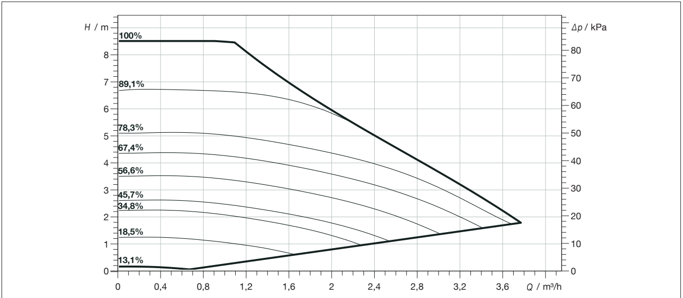
Abb. 36: Kennlinie Wilo Umwälzpumpe (Speicherkreis)
