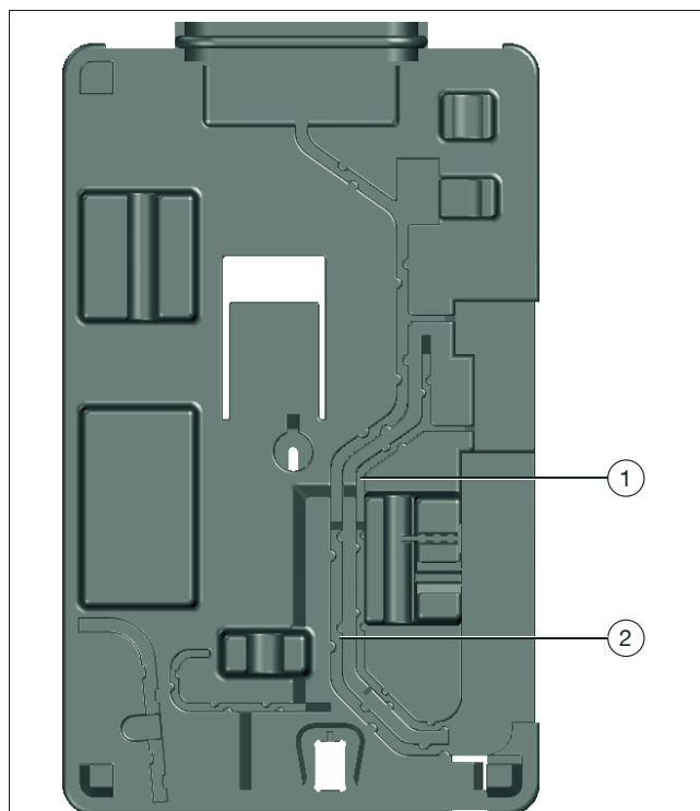
Abb. 19: Kabelkanäle der Unterschale
