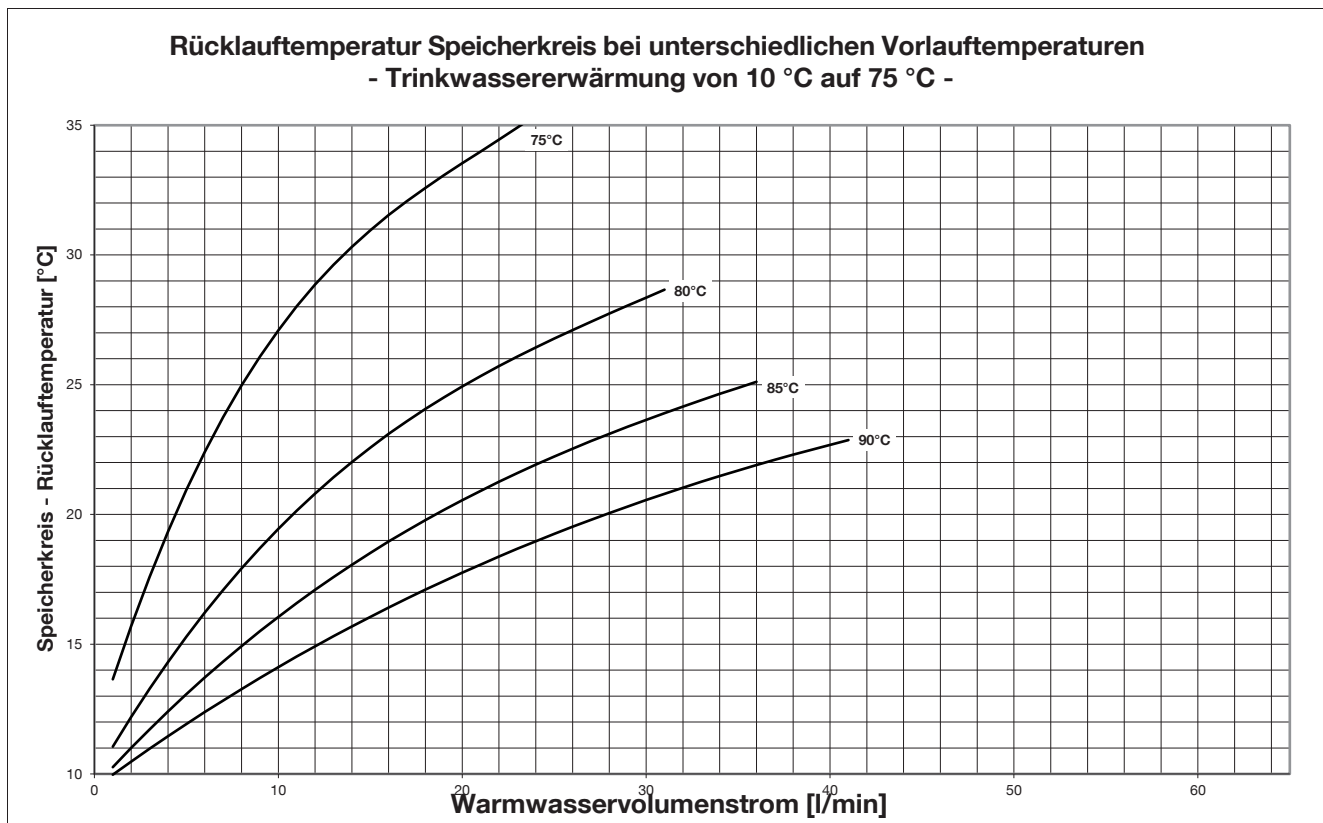
Abb. 52: Rücklauftemperatur Speicherkreis - Trinkwassererwärmung auf 75 °C
