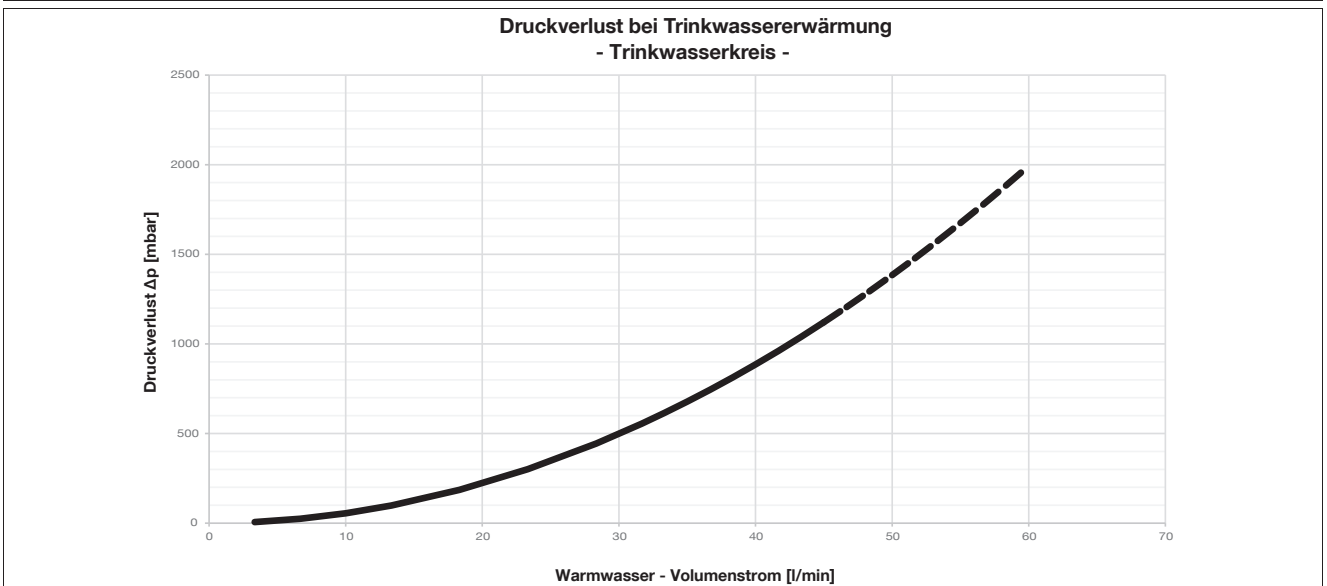
Abb. 38: Kennlinie Druckverlust bei Trinkwassererwärmung (Speicherkreis)
