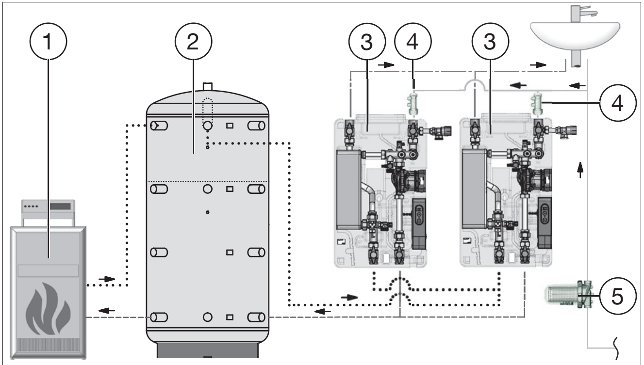
Abb. 3: Anlagenschema mit zwei Frishwasser-Stationen
