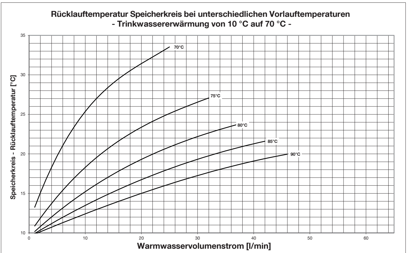
Abb. 50: Rücklauftemperatur Speicherkreis - Trinkwassererwärmung auf 70 °C
