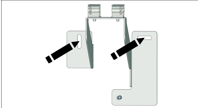
Abb. 10: Wandhalterung als Bohrschablone nutzen
