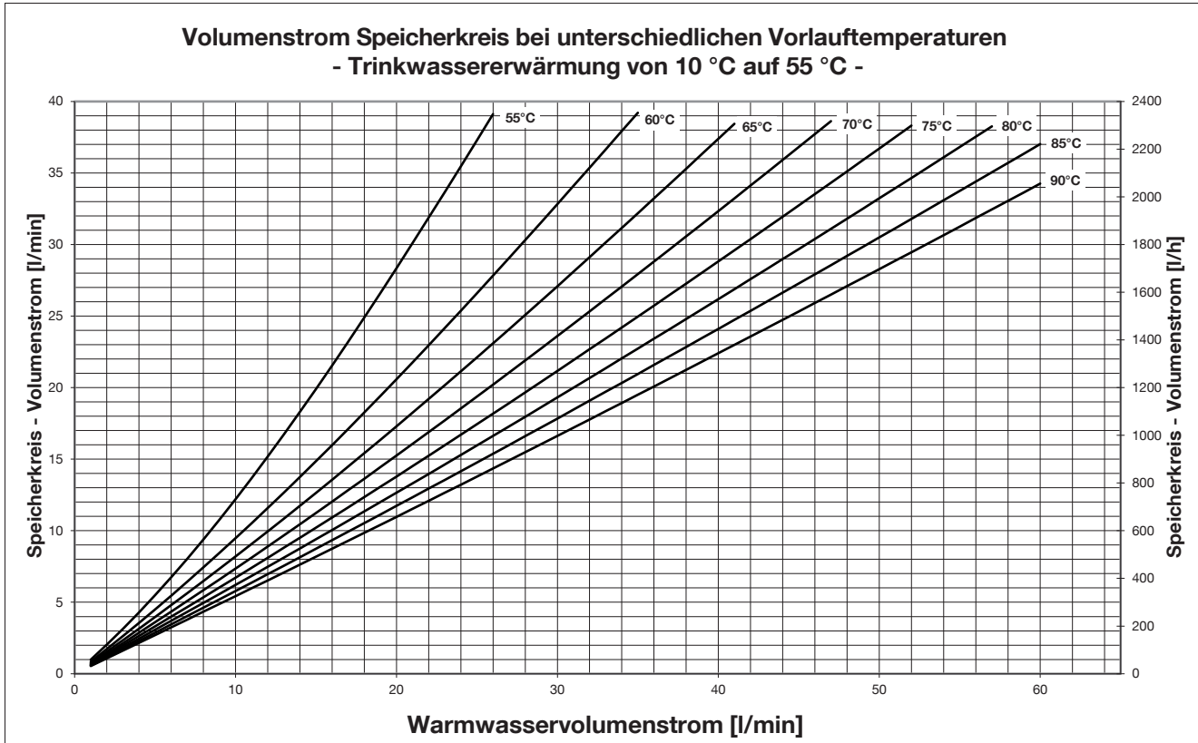
Abb. 43: Volumenstrom Speicherkreis - Trinkwassererwärmung auf 55 °C
