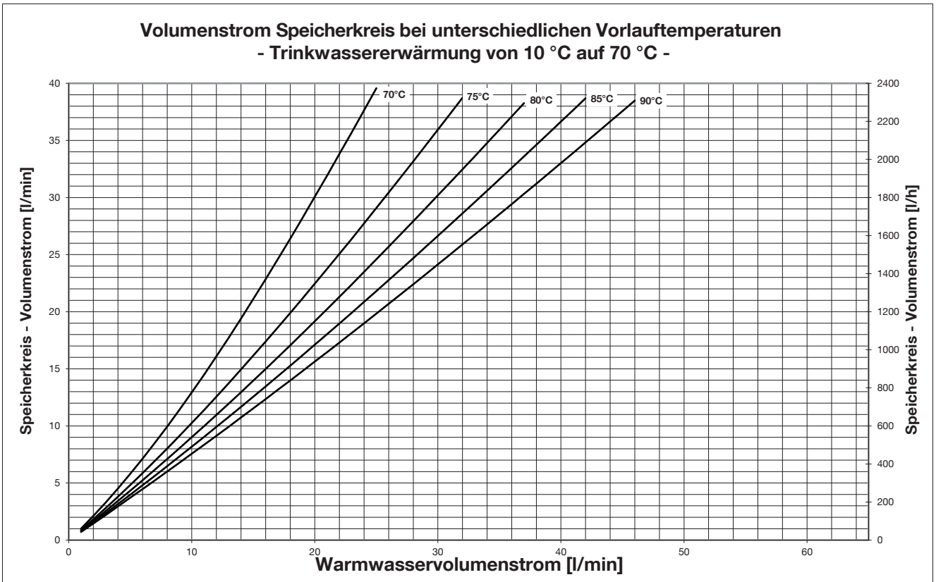
Abb. 49: Volumenstrom Speicherkreis - Trinkwassererwärmung auf 70 °C
