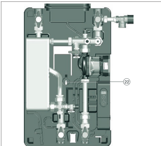
Abb. 11: Position der Unterlegscheibe
