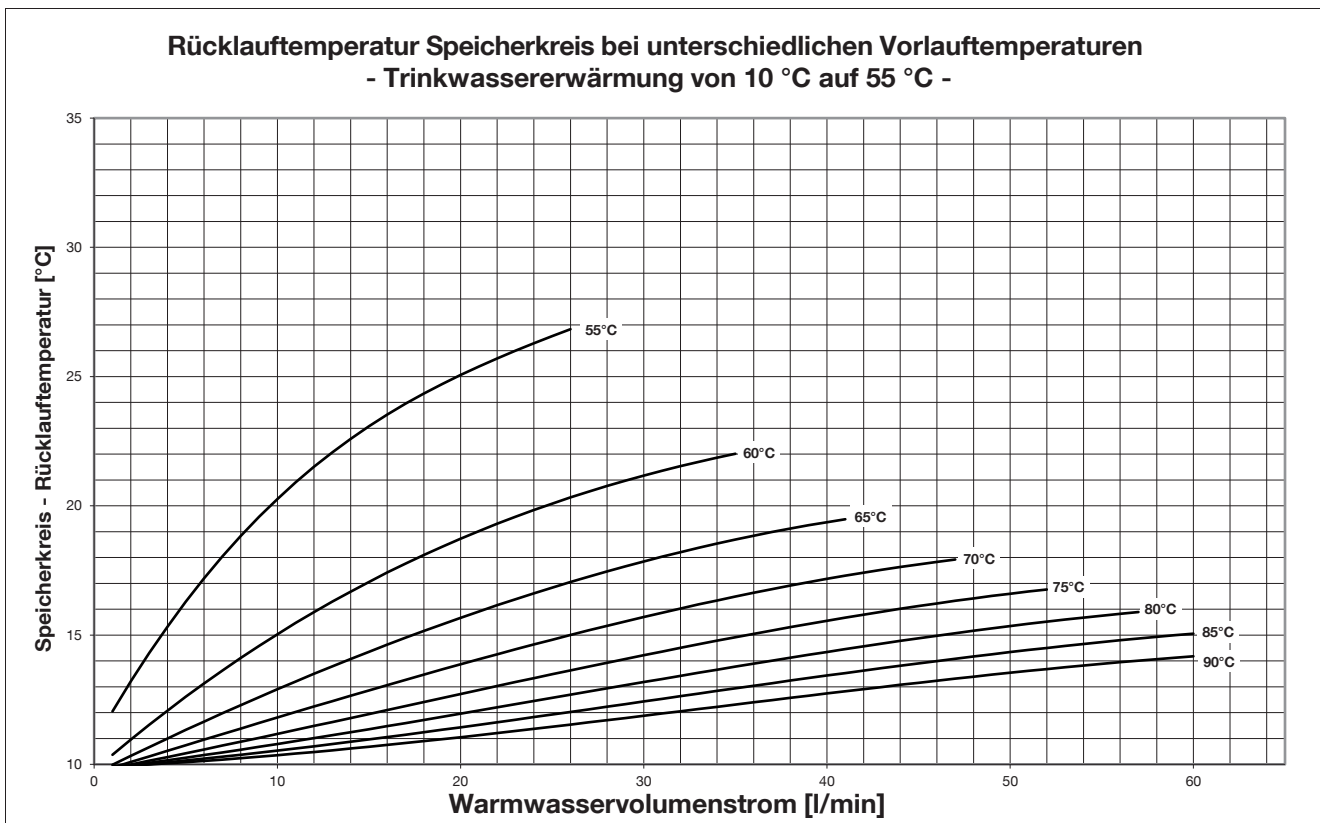
Abb. 44: Rücklauftemperatur Speicherkreis - Trinkwassererwärmung auf 55 °C
