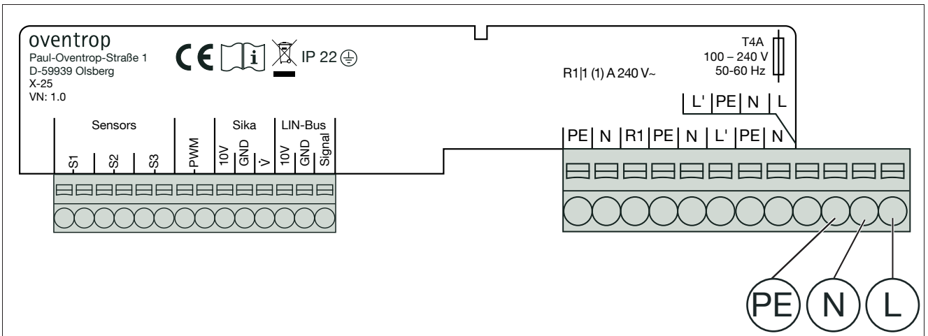
Abb. 7: Klemmbelegung
