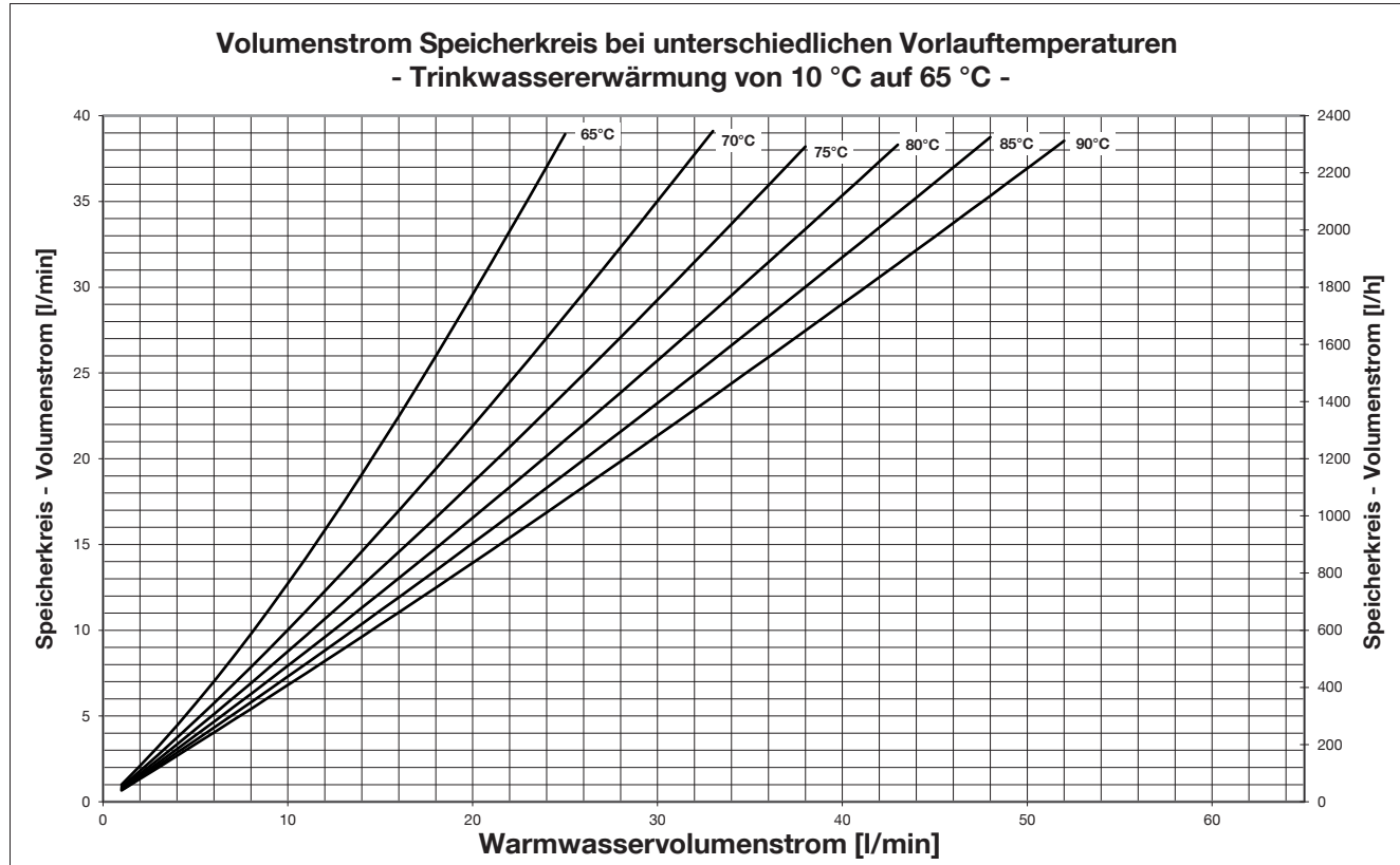
Abb. 47: Volumenstrom Speicherkreis - Trinkwassererwärmung auf 65 °C
