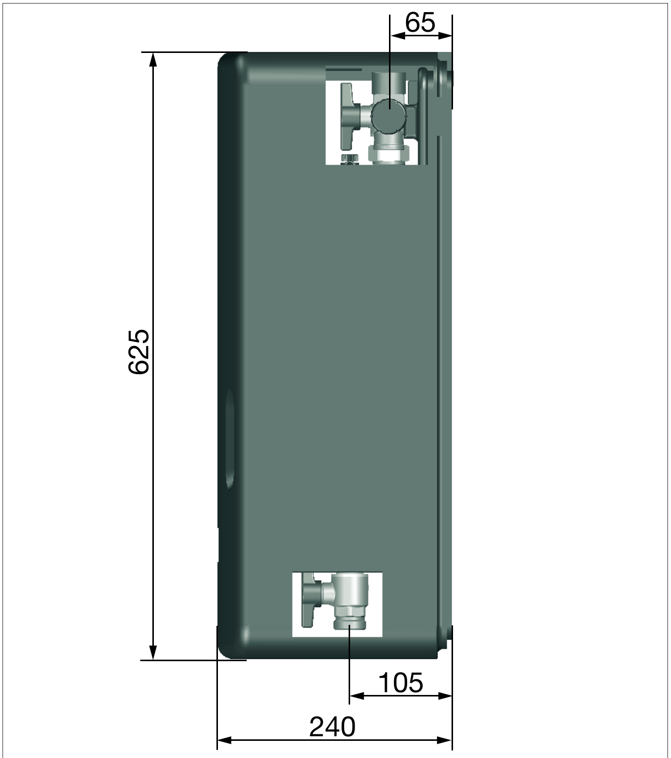
Abb. 5: Abmessungen Frischwasser-Station in mm (Seite)
