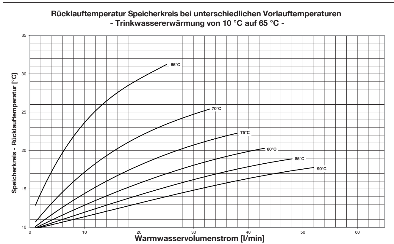
Abb. 48: Rücklauftemperatur Speicherkreis - Trinkwassererwärmung auf 65 °C
