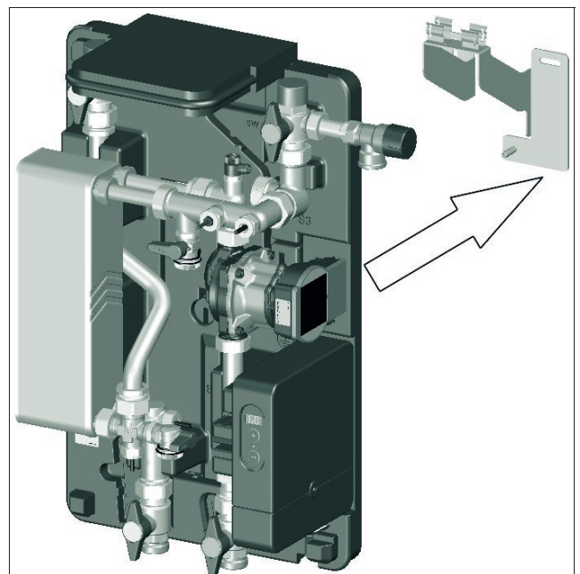
Abb. 9: Wandhalterung demontieren
