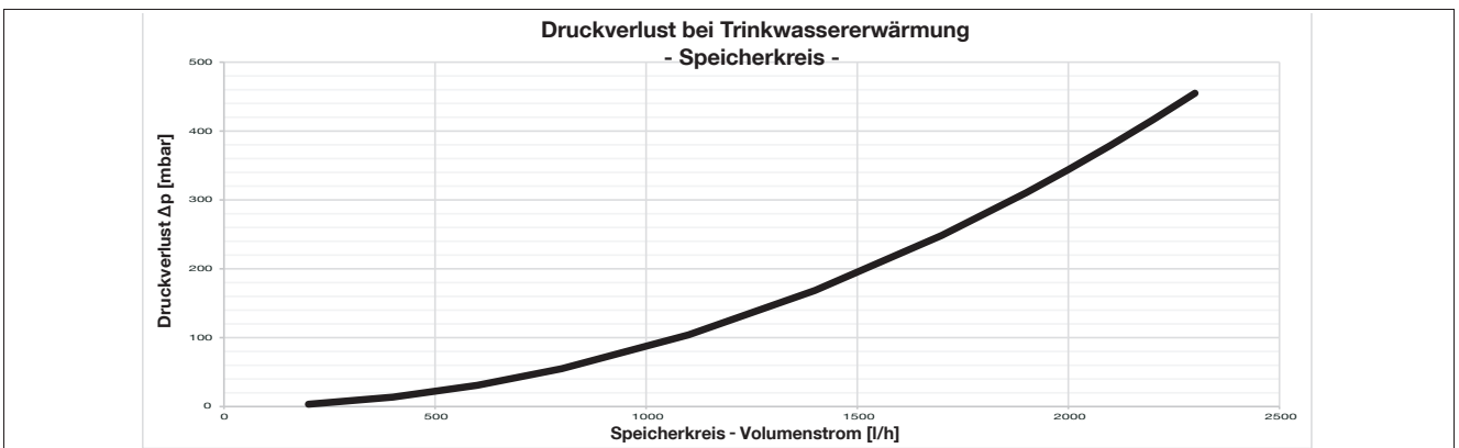
Abb. 37: Kennlinie Druckverlust bei Trinkwassererwärmung (Speicherkreis)
