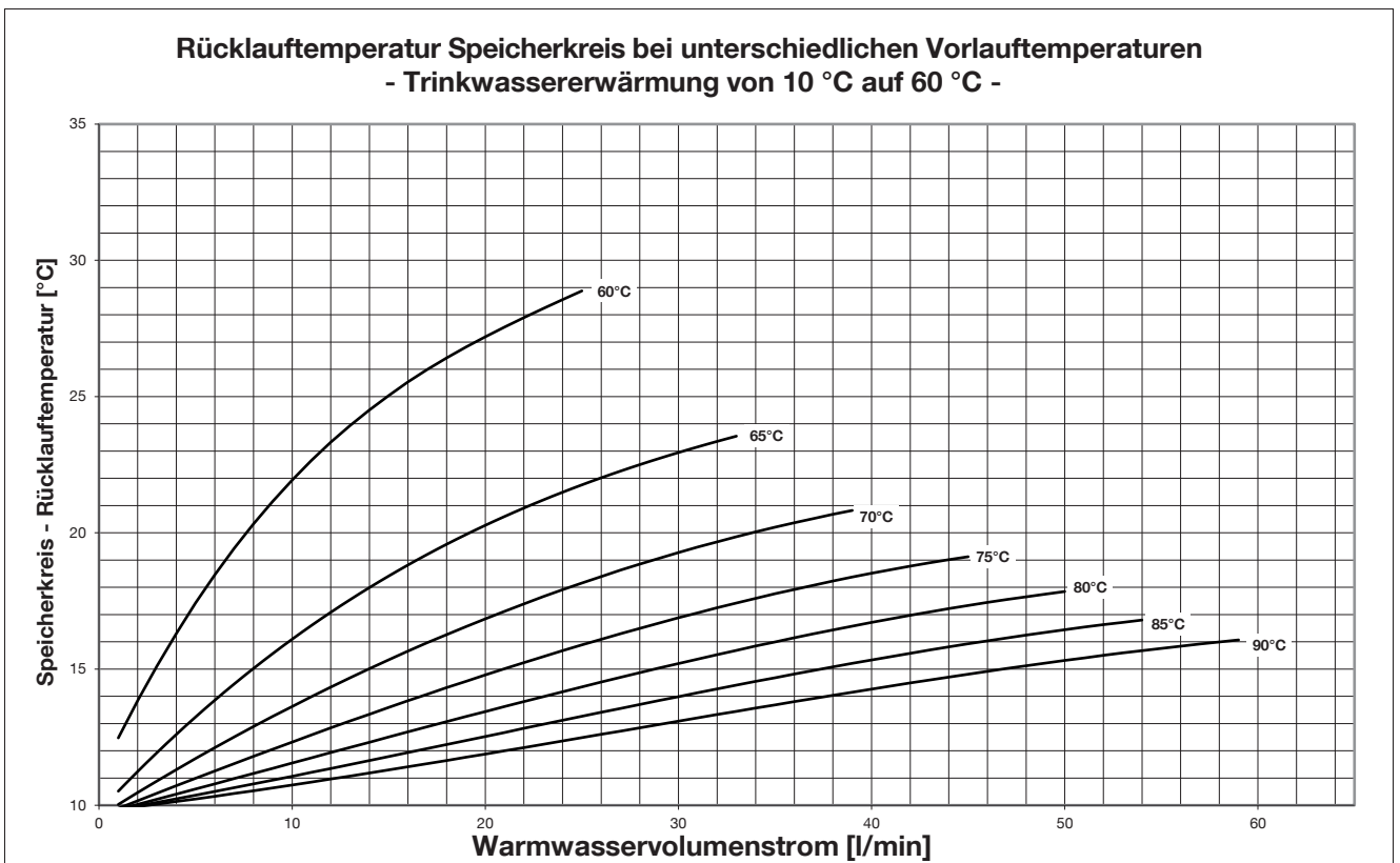
Abb. 46: Rücklauftemperatur Speicherkreis - Trinkwassererwärmung auf 60 °C
