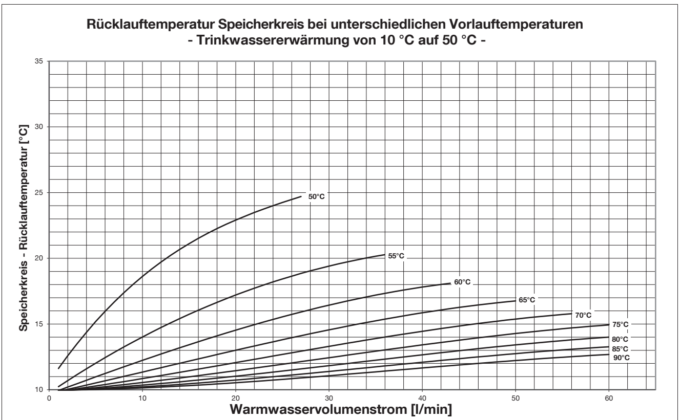
Abb. 42: Rücklauftemperatur Speicherkreis - Trinkwassererwärmung auf 50 °C
