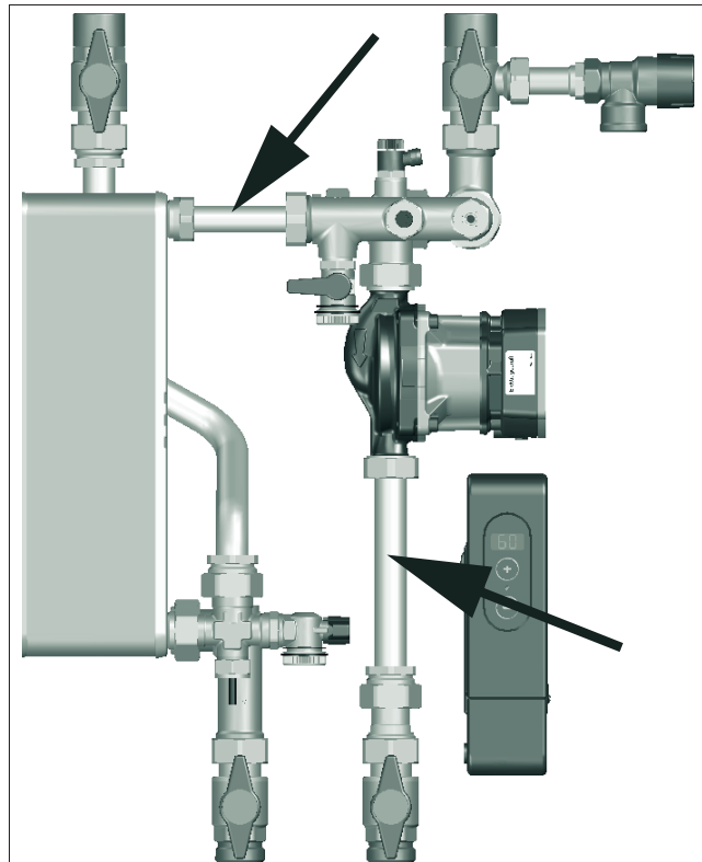
Abb. 13: Potentialausgleich
