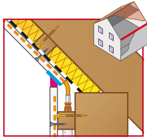
▲ Dachschräge an Kniestock
