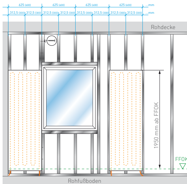
▲ Beispiel CW-Ständerprofilkonstruktion
