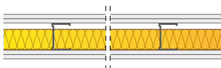
Wandaufbau mit 12,5 mm Fermacell Gipsfaserplatten
